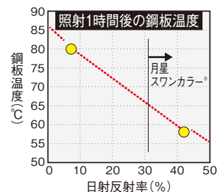
模擬屋根を設置し、赤外線ランプを照射して鋼板温度を測定。
