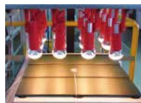
模擬屋根を設置し、赤外線ランプを照射して鋼板温度を測定。
